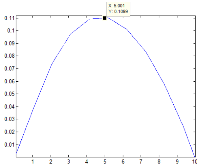
Figure 4.5. Power coefficient ( C_{Pot} ) vs. relação de velocidade de ponta ( \lambda )
